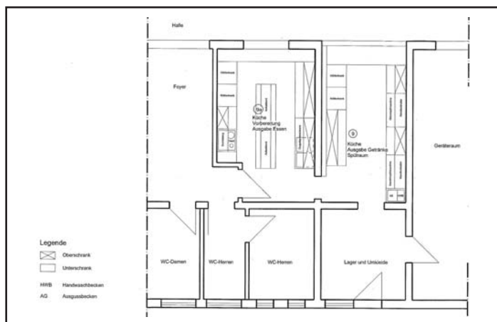
Grundrissplan der geplanten Küchenerweiterung.
